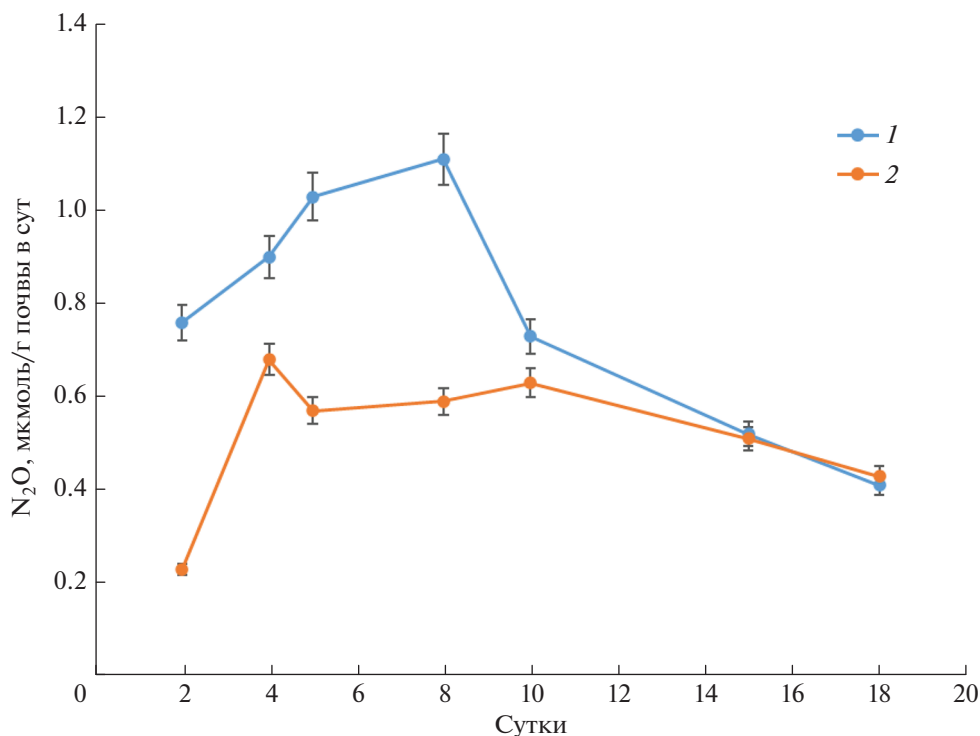
Рис. 2. Влияние хлорида калия на эмиссию N_2O , \mu\text{моль/г} почвы в сутки: 1 – NP, 2 – NP + KCl.
