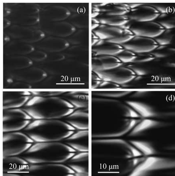
Рис. 4. (Цветной онлайн) Текстура, образованная из холестерика с шагом p = 0.352 \mu\text{м} . Картина напоминает текстуру конфокальных доменов в смектических жидких кристаллах. Отражение (а), пропускание (б)–(д), поляризаторы скрещены. Домены могут образовывать пространственно упорядоченные группы (с). (д) – Два домена показаны в увеличенном масштабе
