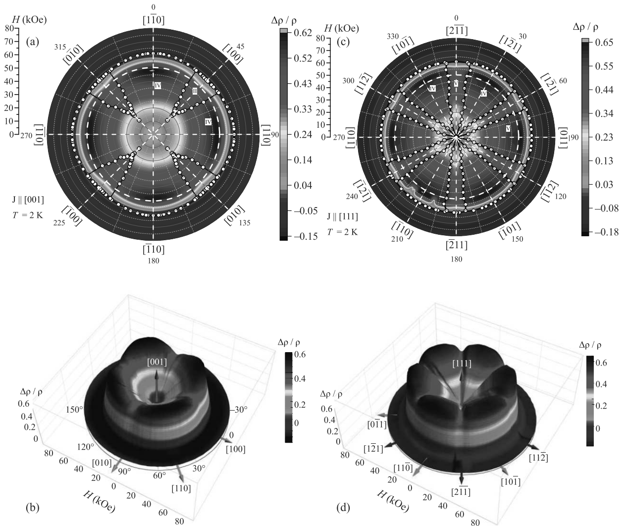
Рис. 2. (Цветной онлайн) Магнетосопротивление \Delta\rho/\rho = f(H, \varphi) в \text{Er}^{11}\text{B}_{12} при T = 2\text{ K} в полярных (а), (с) и цилиндрических (b), (d) координатах для направлений тока \mathbf{I} \parallel [001] и \mathbf{I} \parallel [111] , соответственно. Римскими цифрами показаны разные магнитные фазы в АФ состоянии (сохранена нумерация фаз [28], см. также рис. S2 в дополнительных материалах). Белый пунктир при H = 50\text{ кЭ} показывает сферу, для которой на рис. 3b представлен контур сечения магнитных фаз построенной 3D H-\varphi-\theta фазовой диаграммы
