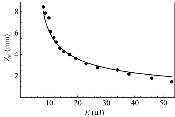
Рис. 3. Расстояние до начала филаментации z_{\text{фн}} аксиально-несимметричного оптического вихря в кристалле LiF в зависимости от энергии импульса (точки, эксперимент). Расстояние до нелинейного фокуса, вычисленное по формуле Марбургера для фокусированного на 1 \text{ см} гауссова пучка радиусом r_0 = 58 \text{ мкм} (сплошная кривая)
