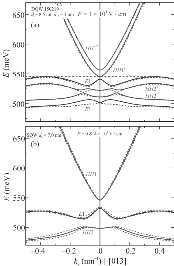
Рис. 7. (Цветной онлайн) (а) – Спектр ДКЯ в перпендикулярном электрическом поле F = 1 \times 10^4 В/см. Сплошные и штриховые линии для разных ориентаций спина. (б) – В спектре одиночной квантовой ямы шириной 7 нм также имеется тонкий баланс между ЦМ и БМ. Но поле F на него практически не влияет. Здесь сплошные линии без поля, а штриховые – спектр в поле F = 4 \times 10^4 В/см. Изменения проявляются только в виде слабо выраженного эффекта Рашбы – в небольшом расщеплении по спину вследствие перекося ямы
