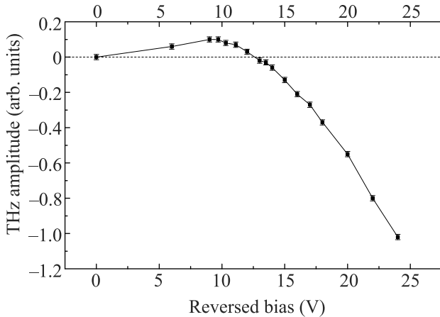
Рис. 4. Зависимость амплитуды основного импульса ТГц излучения от напряжения обратного смещения на структуре СЭ на основе a-Si:H/a-SiC:H/c-Si
