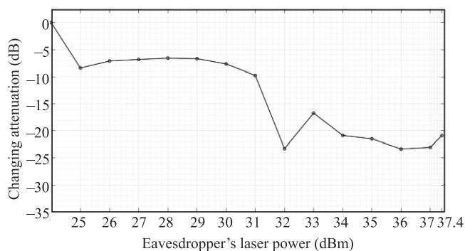
Рис. 5. (Цветной онлайн) Изменение ослабления светофильтра #3 относительно начального значения
