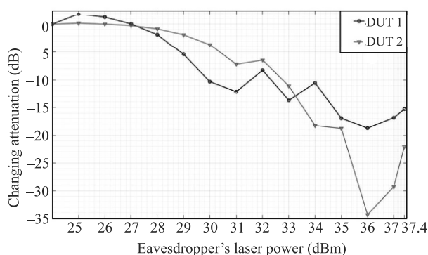
Рис. 3. (Цветной онлайн) Изменение ослабления светофильтров #1, 2 относительно начального значения
