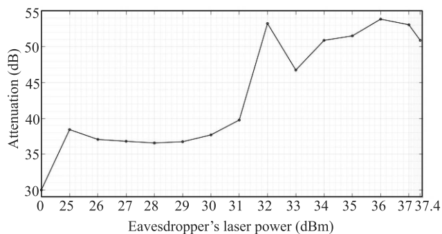
Рис. 4. (Цветной онлайн) Ослабление светофильтра #3 в зависимости от мощности атакующего излучения
