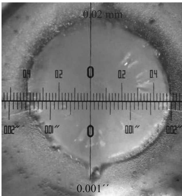
Рис. 6. (Цветной онлайн) Кратер в масштабе
