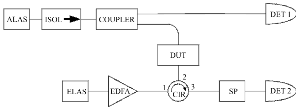
Рис. 1. Экспериментальная схема измерения. ALAS – контрольный лазер; ISOL – изолятор для мощного лазерного излучения; COUPLER – светоделитель 90/10; DET1 – измеритель мощности # 1 для детектирования излучения контрольного лазера; DUT – исследуемый образец; ELAS – атакующий лазер, EDFA – усилитель лазерного излучения; CIR – циркулятор (цифрами обозначены порты); SP – спектральный фильтр; DET2 – измеритель мощности # 2 для детектирования излучения контрольного лазера; прошедшего через образец
