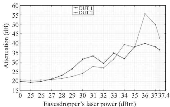
Рис. 2. (Цветной онлайн) Ослабления светофильтров #1, 2 в зависимости от мощности атакующего излучения
