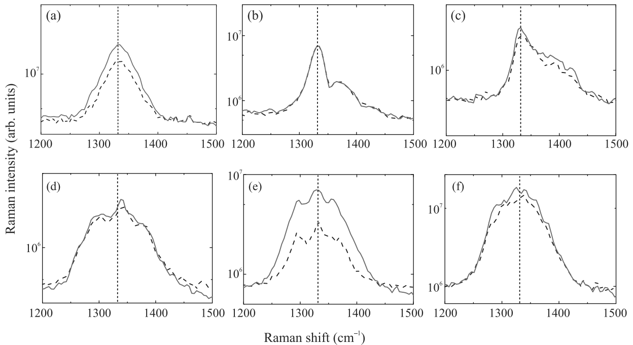
Рис. 2. (Цветной онлайн) Характерные спектры КР-сигнала центрального оптического фотона алмаза для различных длительностей УКИ: 0.3 (a), 0.69 (b), 1.3 (c), 2.3 (d), 6.3 (e) и 12 (f) пс. Цветами показаны спектры для разных значений пиковой плотности энергии УКИ: 0.16 (темно-синяя штриховая кривая) и 0.32 (светло-серая кривая) Дж/см 2 . Пунктирная линия показывает центр линии фона 1332 см -1
