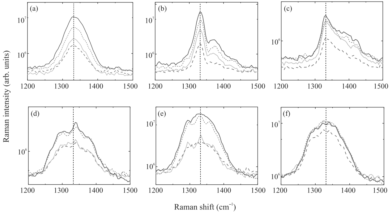
Рис. 1. (Цветной онлайн) Характерные спектры КР-сигнала центрального оптического фотона алмаза для различных длительностей УКИ: 0.3 (а), 0.69 (б), 1.3 (с), 2.3 (д), 6.3 (е) и 12 (ф) пс. Цветами показаны спектры для разных падающих пиковых интенсивностей УКИ: 0.03 (темно-серая штрихованная кривая), 0.06 (светло-серая кривая), 0.12 (оранжевая пунктирная кривая), 0.24 (бордовая кривая) ТВт/см 2 . Пунктирная линия показывает центр линии фонона 1332 см -1
