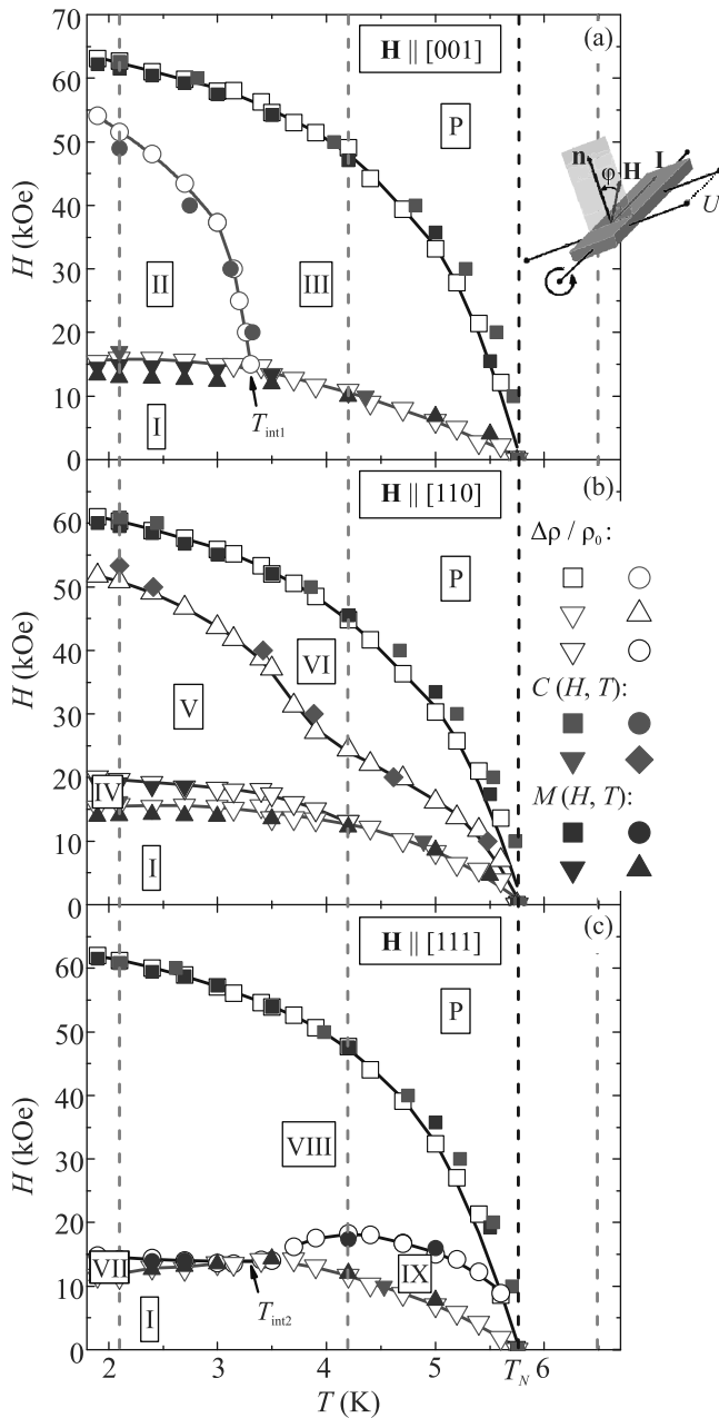
Рис. 1. (Цветной онлайн) Магнитные фазовые H – T диаграммы \text{Ho}_{0.8}\text{Lu}_{0.2}\text{B}_{12} для направлений нормали (a) – \mathbf{n}||[001] , (b) – \mathbf{n}||[110] и (c) – \mathbf{n}||[111] , полученные из данных магнетосопротивления, теплоемкости и намагниченности [11]. Вертикальными пунктирными прямыми отмечена T_N и температуры, при которых регистрировались угловые кривые холловского сопротивления. Римскими цифрами обозначены магнитоупорядоченные фазы, P – парамагнитная фаза
