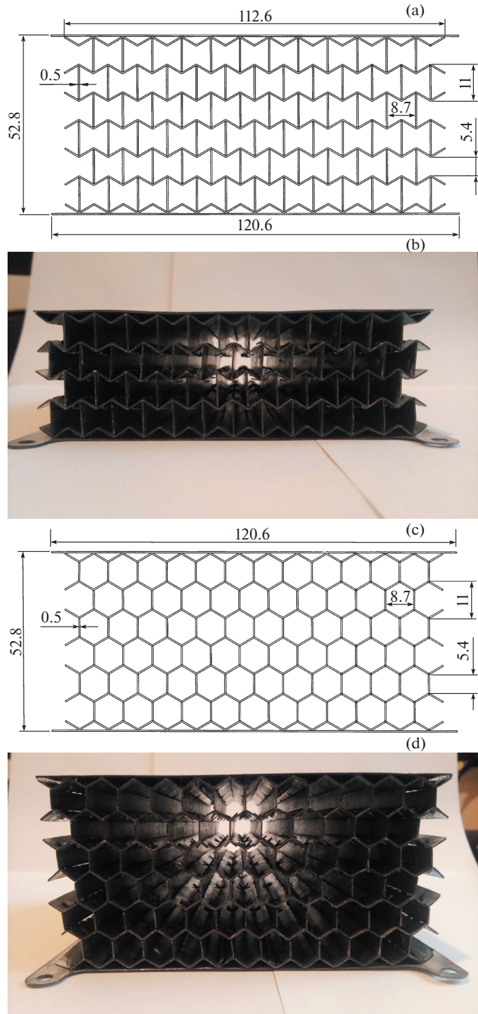
Рис. 1. Внутренняя структура образцов метаматериалов и их геометрические размеры в мм: (а), (b) – акустический; (с), (d) – неакустический сотовые образцы.
