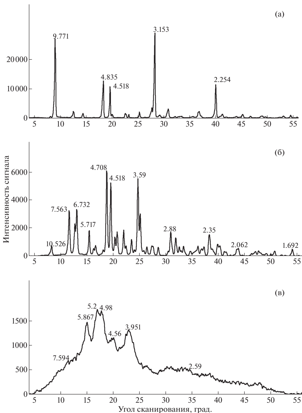
Рис. 1. Порошковые рентгеновские диффрактограммы: глюкозы (а); сахарозы (б); крахмала (в).
