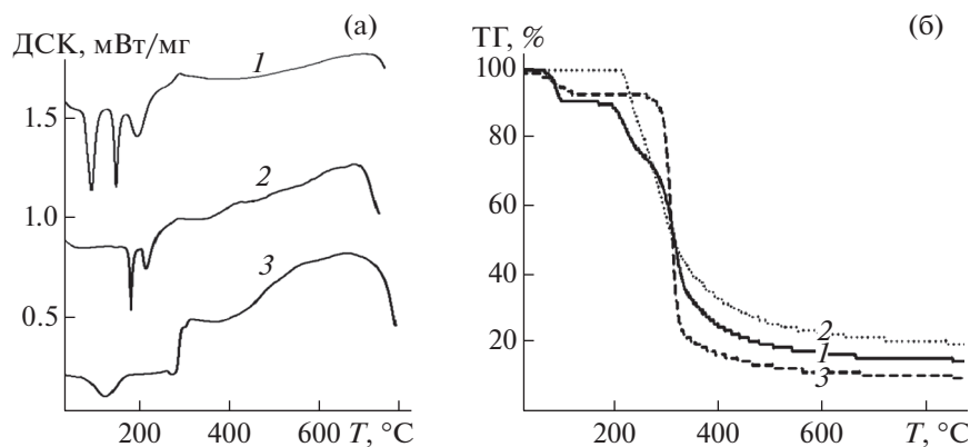
Рис. 2. Кривые дифференциально-сканирующей калориметрии (а) и потери массы (б) при термическом анализе глюкозы (1), сахарозы (2), крахмала (3) в аргоне.
