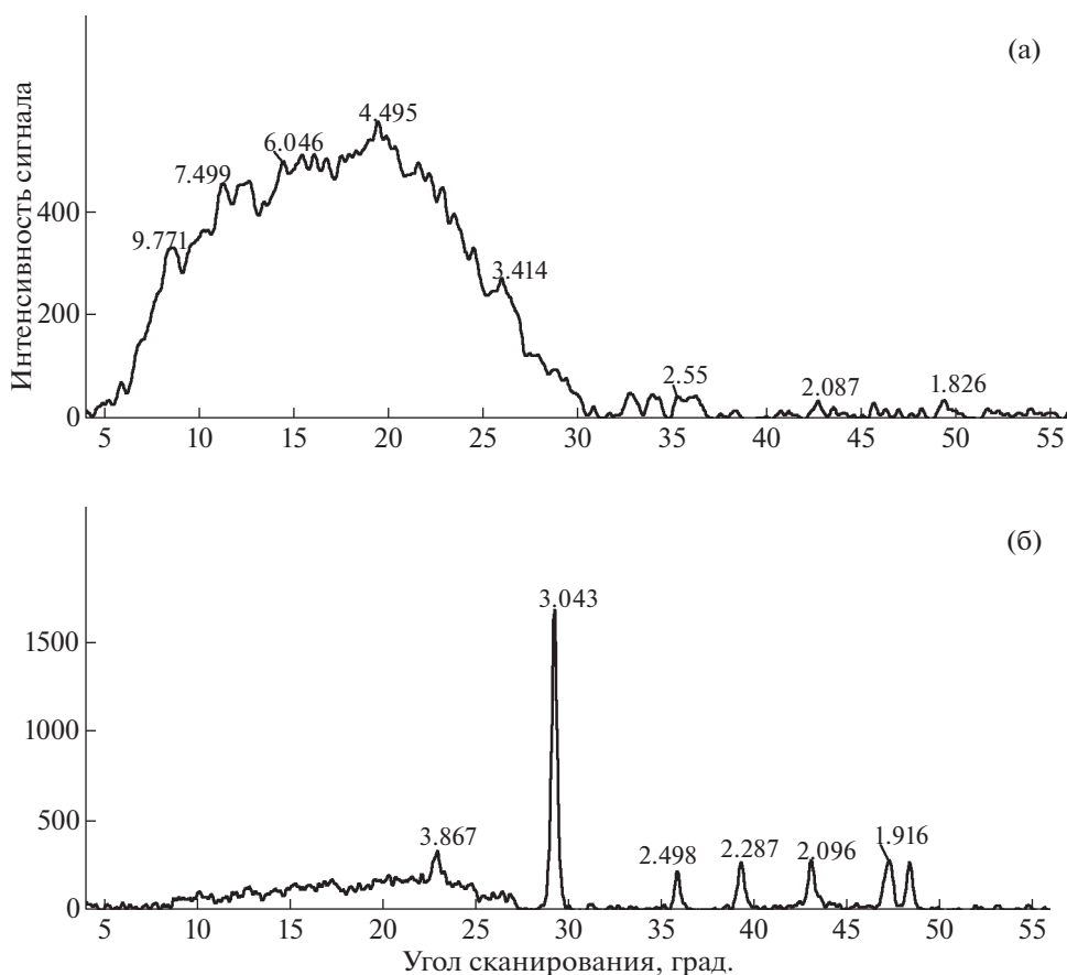
Рис. 3. Порошковые рентгеновские дифрактограммы углерода из сахарозы с добавками хлоридов кальция (а) и железа (б).
